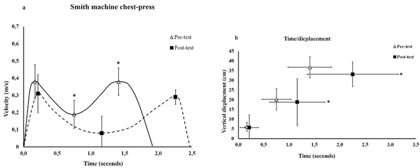
Figura 3. Los cambios medios \pm SD en la velocidad de la barra (a), el tiempo de levantamiento y el desplazamiento de la barra (b), antes y después del entrenamiento en el grupo de máquina Smith en el ejercicio entrenado. * significativamente diferente al pre-test ( p < 0.05 ).
